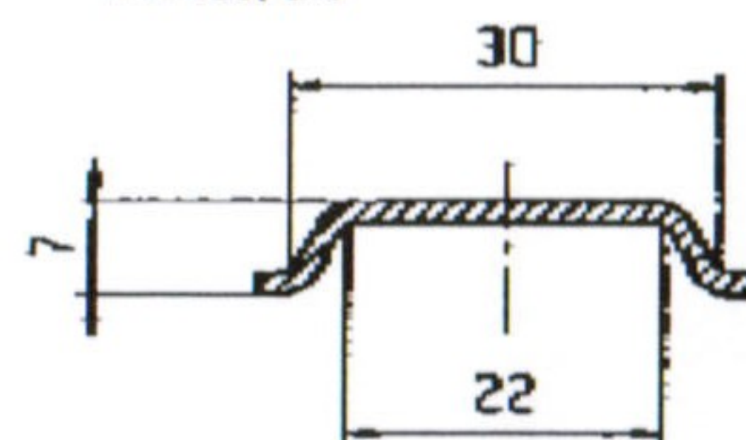
AA断面
