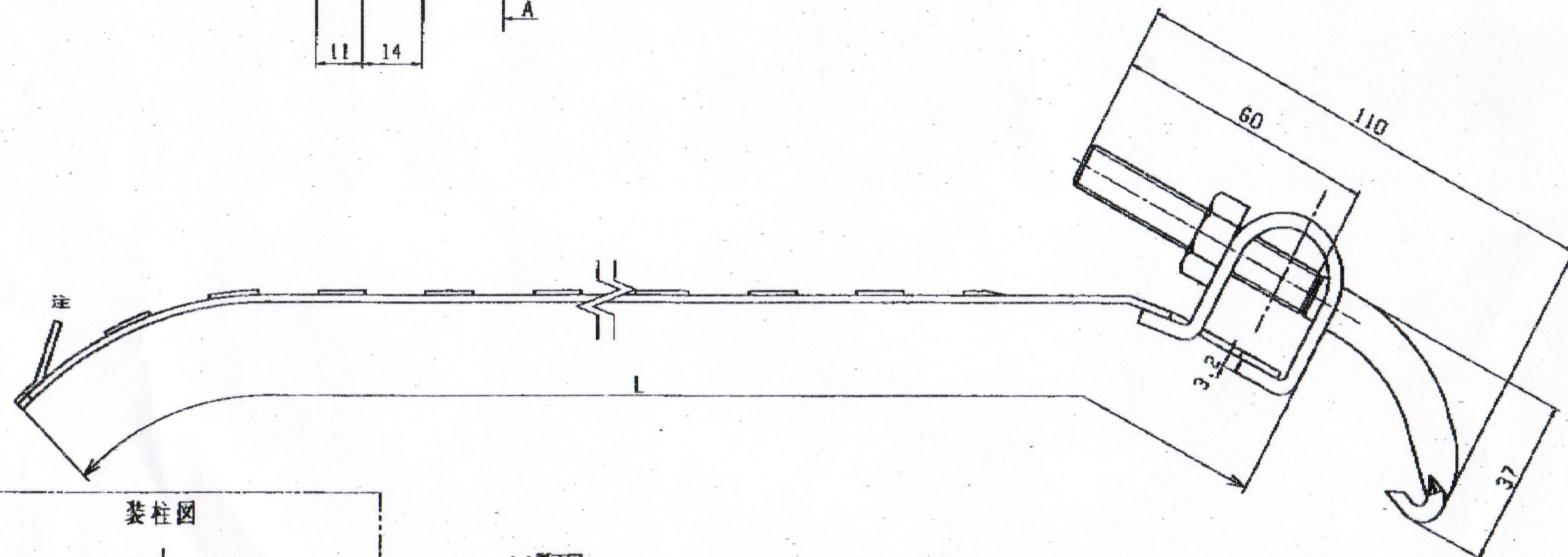
AA断面図
