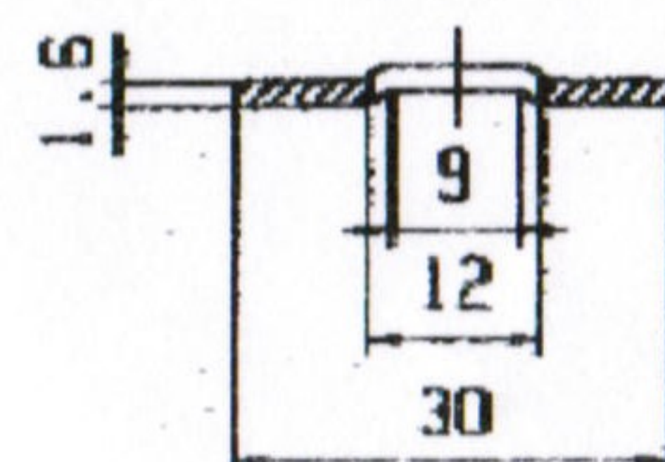
AA断面図
