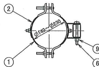
A-A矢視図
