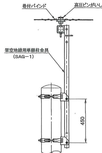
使用状態例
