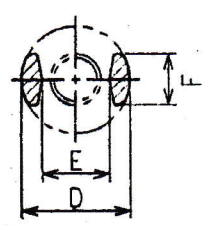
断面 a-a
